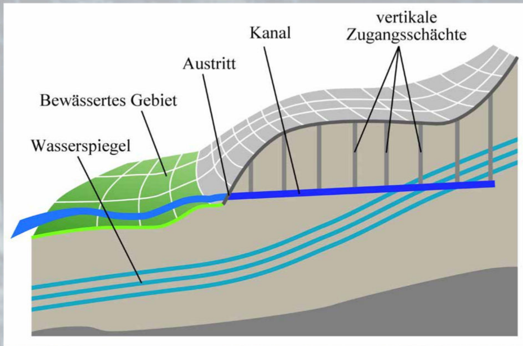
Abb.: nach https://commons.wikimedia.org/w/index.php?curid=5824544 Funktionsschema eines puquio .
